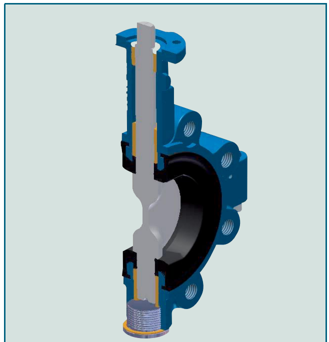
Klapka Z614-A v řezu
